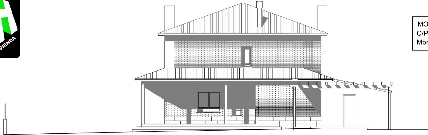
ALZADO LATERAL
